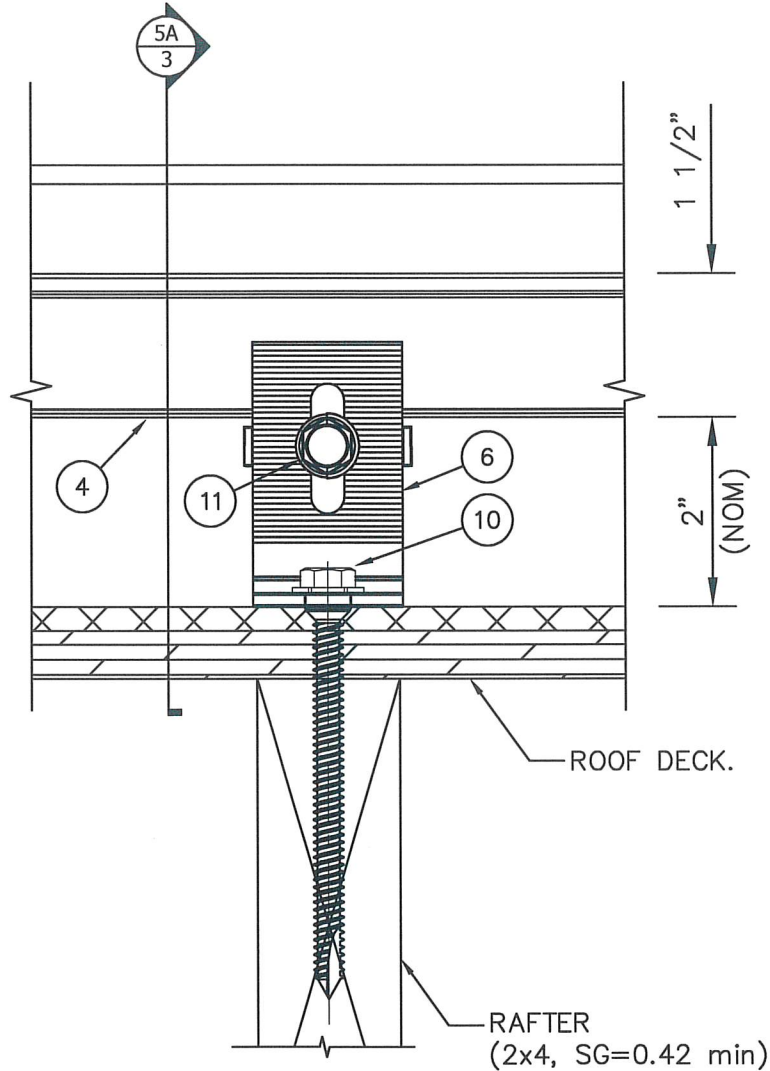
2 2 L-FOOT DETAIL
